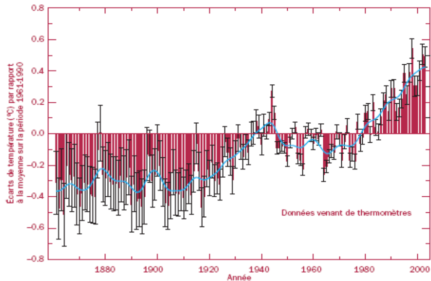
Figure 3. Variations de la température moyenne observée à la surface du globe depuis 1861 (source : Hadley Centre)
